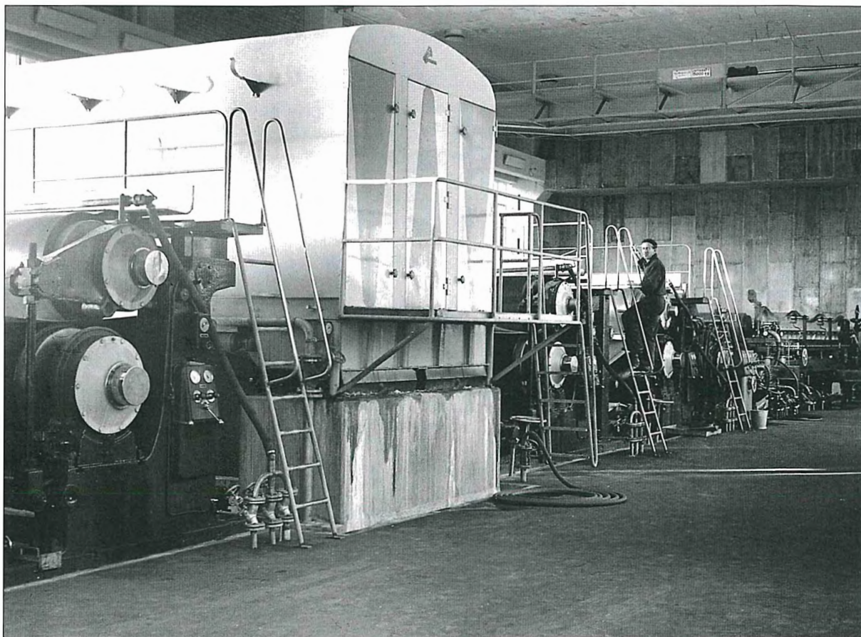
Interiörbild från Edsvalla sulfittfabrik, ett av Mölnbacka-Trysils bruk. Foto: Lindgrens foto, 1958. Ur Uddeholms bildarkiv, volym 56.
